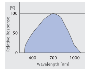
Pyranometer ML-020VM
